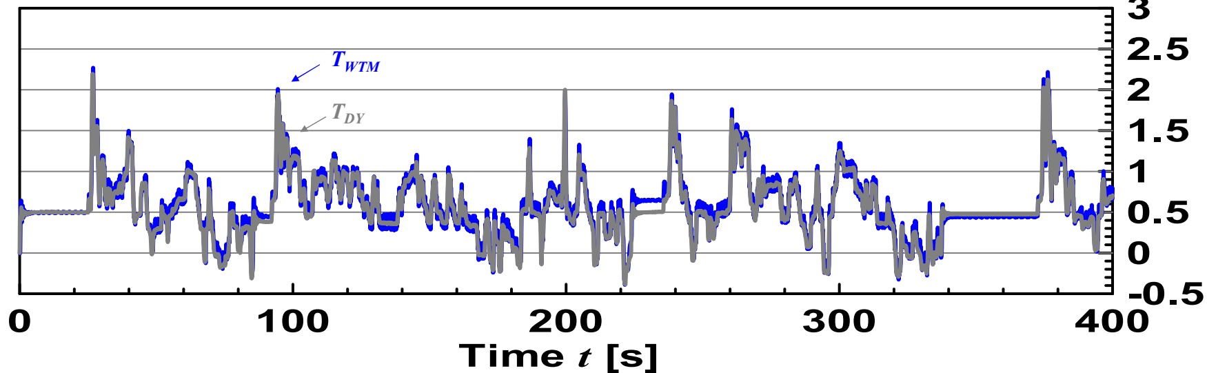
シャーシダイナモ走行データ (JC08)
